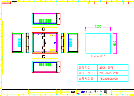
리프트(영사대, 전개도)
