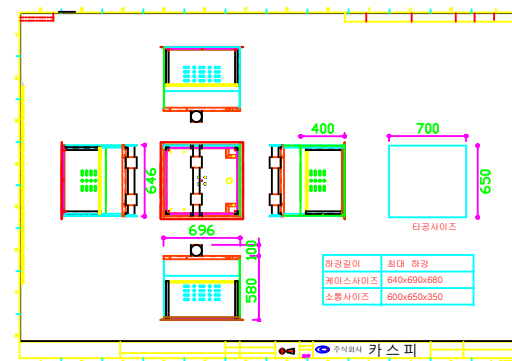
리프트(영사대). 전개도
